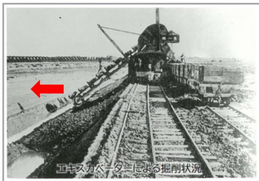
▲エキスカベーターの写真 出典 国土交通省 荒川下流河川事務所
